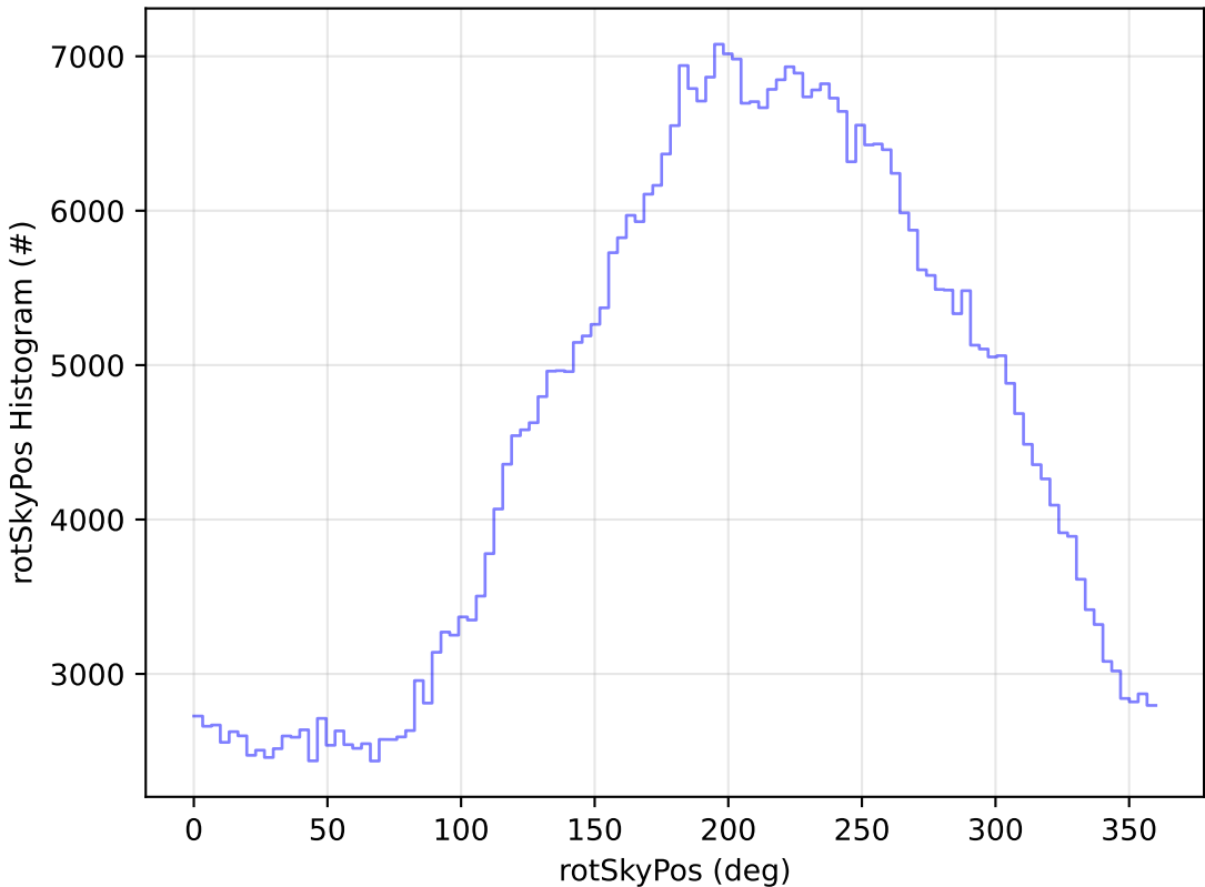
weather_cloudso0v3.4_10yrs WFD i band: rotSkyPos Histogram
