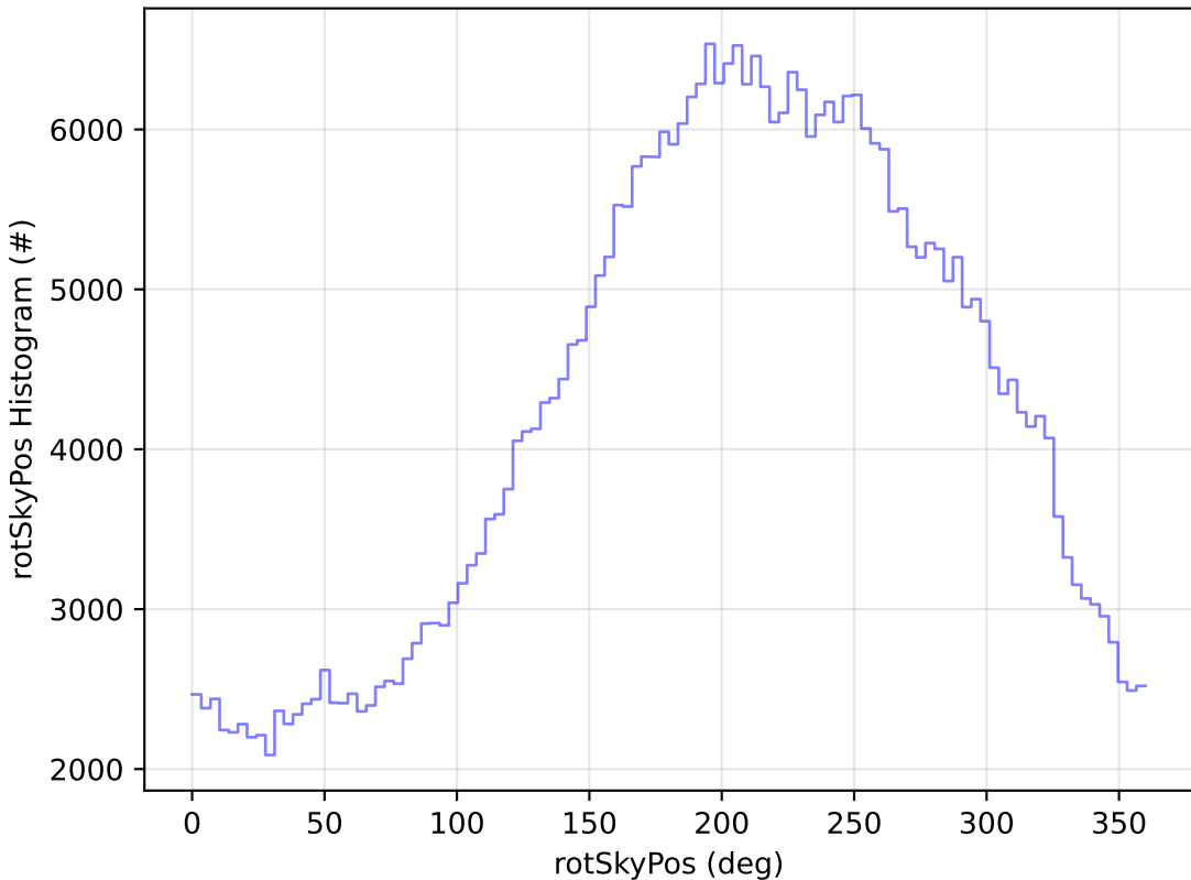
weather_cloudso0v3.4_10yrs All sky z band: rotSkyPos Histogram
