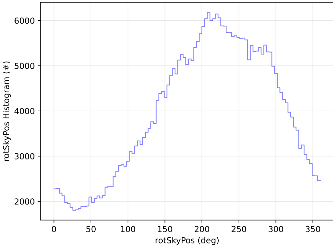
weather_cloudso0v3.4_10yrs All sky y band: rotSkyPos Histogram
