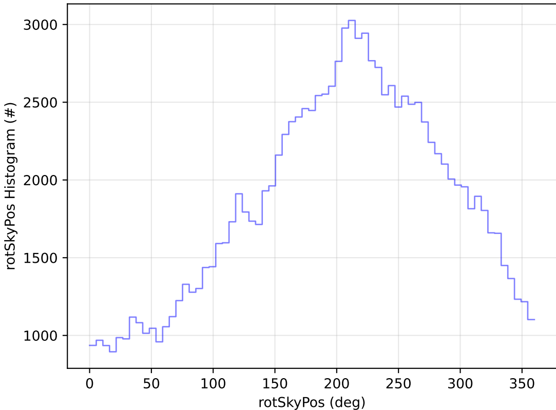
weather_cloudso0v3.4_10yrs All sky u band: rotSkyPos Histogram
