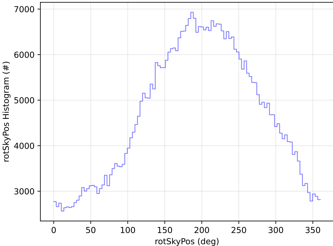
weather_cloudso0v3.4_10yrs All sky r band: rotSkyPos Histogram
