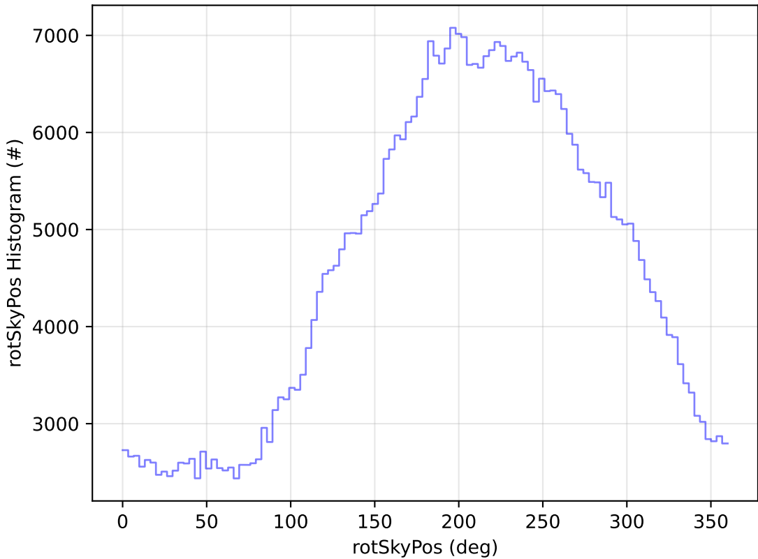
weather_cloudso0v3.4_10yrs All sky i band: rotSkyPos Histogram
