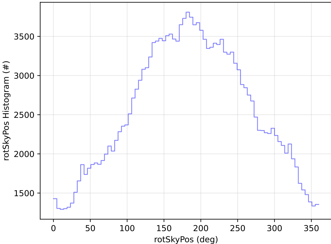
weather_cloudso0v3.4_10yrs All sky g band: rotSkyPos Histogram
