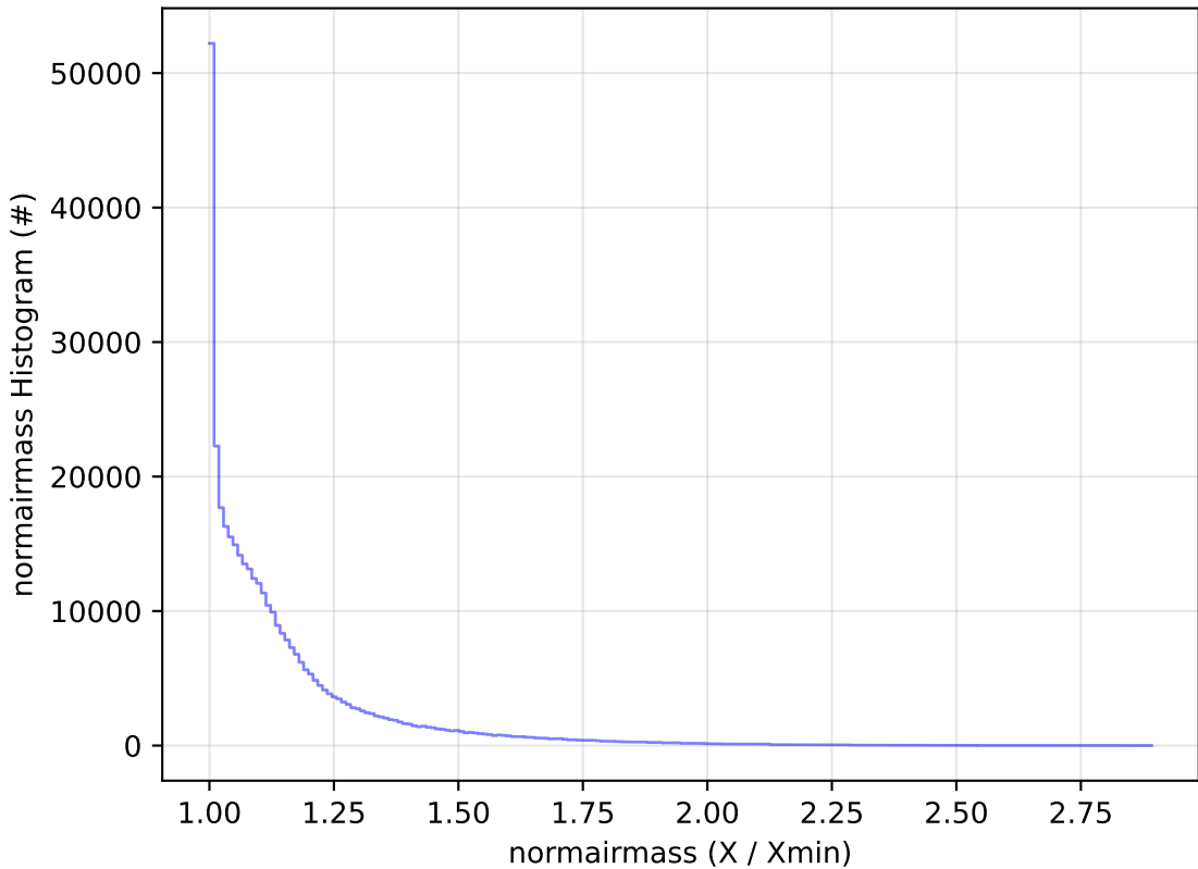
weather_cloudso0v3.4_10yrs WFD y band: normairmass Histogram
