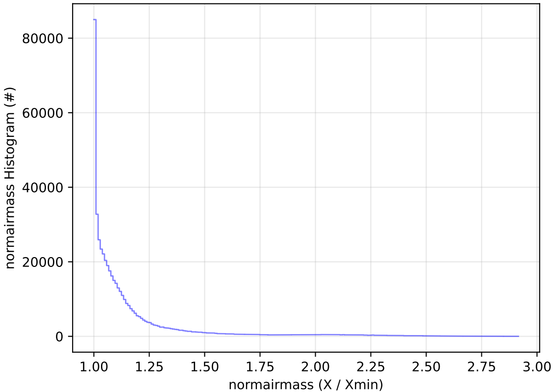
weather_cloudso0v3.4_10yrs WFD i band: normairmass Histogram
