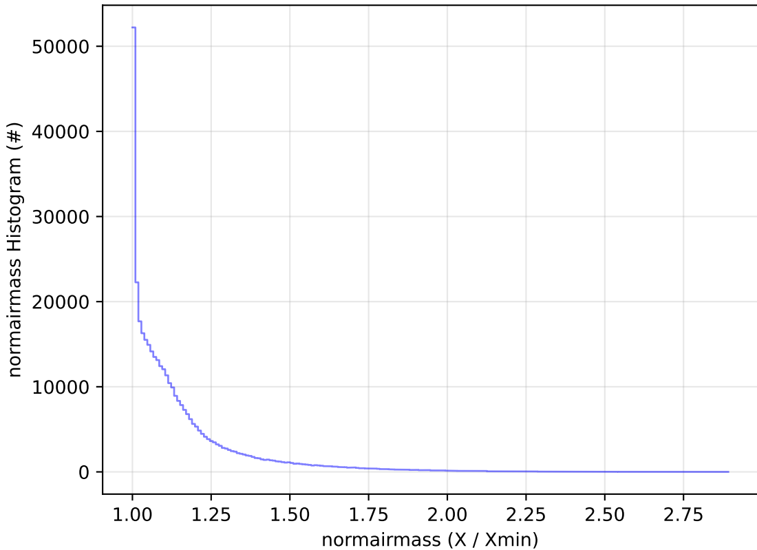
weather_cloudso0v3.4_10yrs All sky y band: normairmass Histogram
