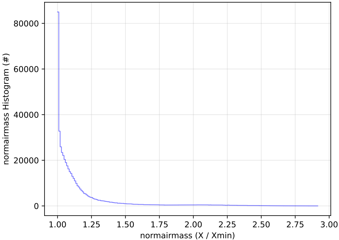
weather_cloudso0v3.4_10yrs All sky i band: normairmass Histogram
