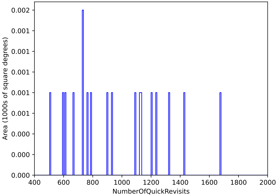
weather_cloudso0v3.4_10yrs WFD: NumberOfQuickRevisits
