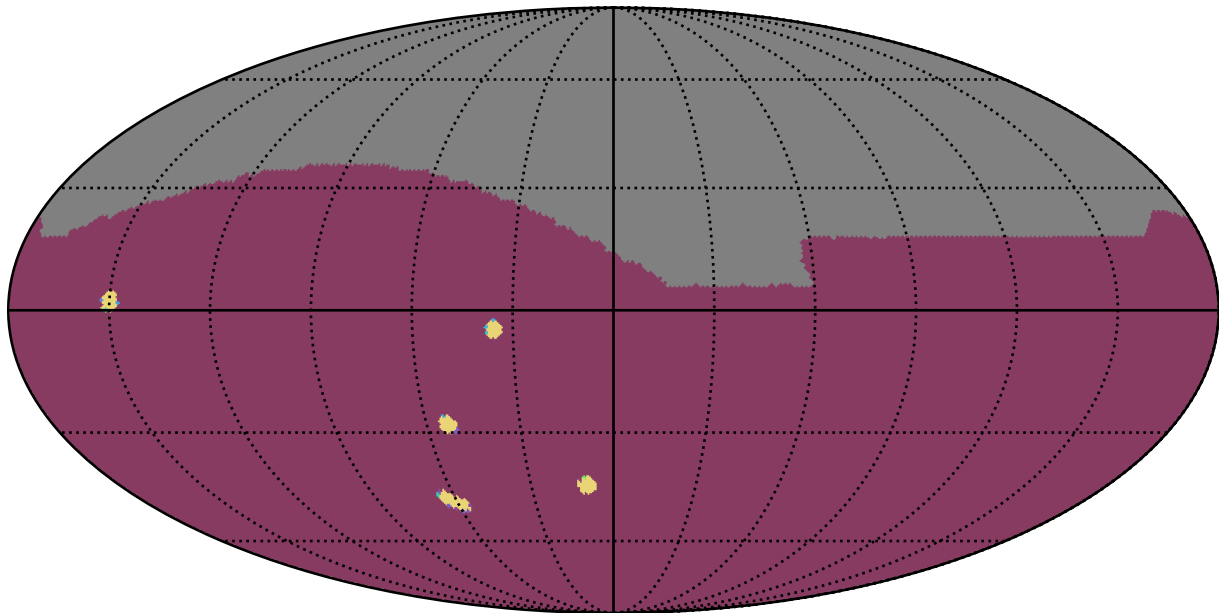
weather_cloudso0v3.4_10yrs All sky: NumberOfQuickRevisits
