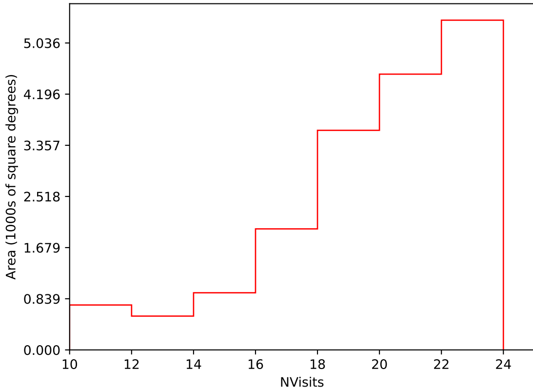
weather_cloudso0v3.4_10yrs Yr 1 i band: NVisits
