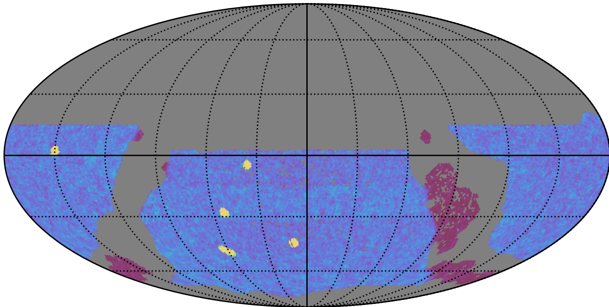
weather_cloudso0v3.4_10yrs WFD y band: NVisits
