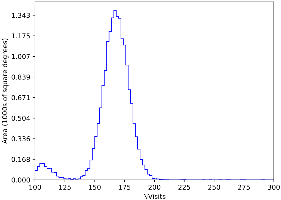
weather_cloudso0v3.4_10yrs WFD y band: NVisits
