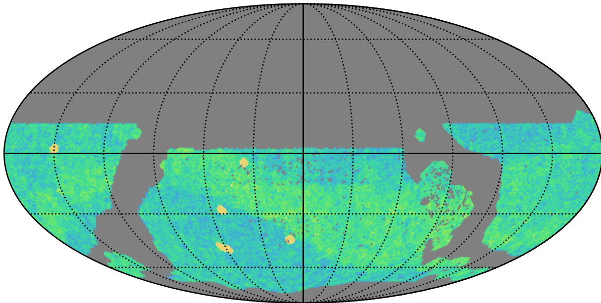
weather_cloudso0v3.4_10yrs WFD i band: NVisits
