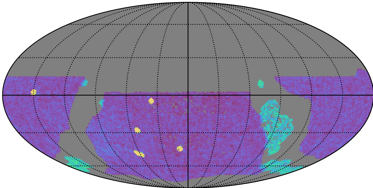
weather_cloudso0v3.4_10yrs WFD g band: NVisits
