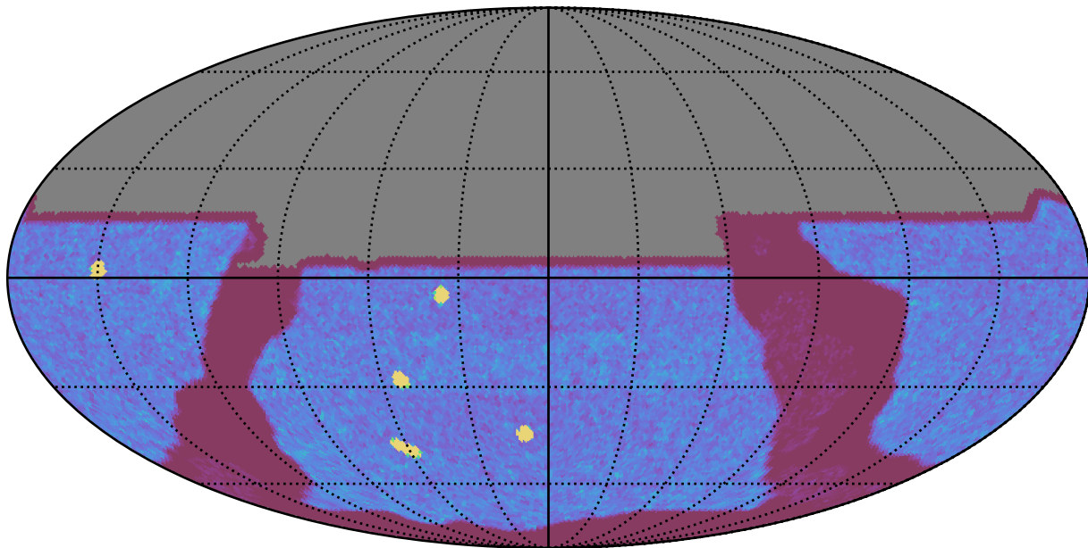
weather_cloudso0v3.4_10yrs All sky y band: NVisits
