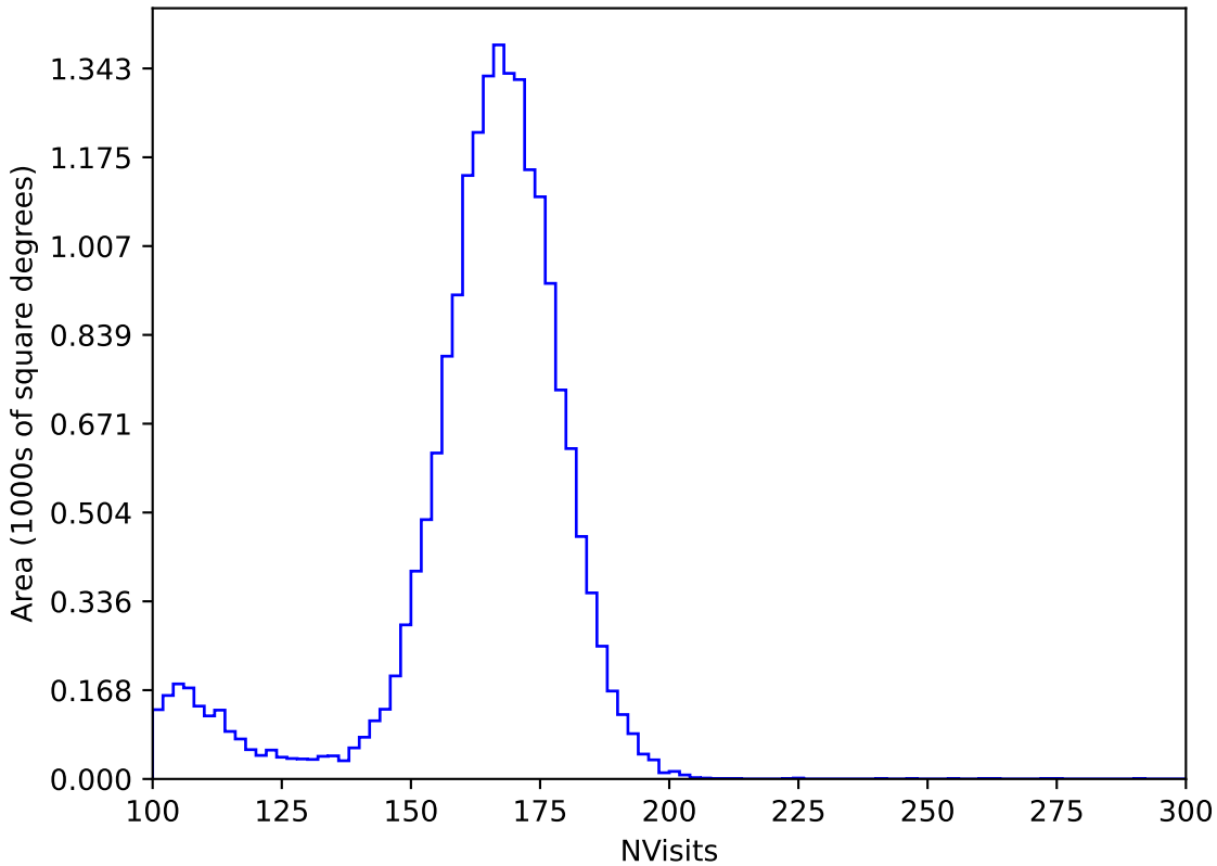
weather_cloudso0v3.4_10yrs All sky y band: NVisits
