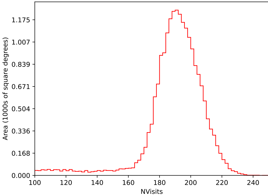
weather_cloudso0v3.4_10yrs All sky i band: NVisits
