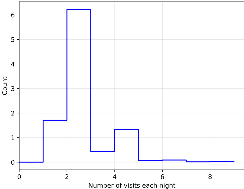
1e6 weather_cloudso0v3.4_10yrs All sky: NVisitsPerNight
