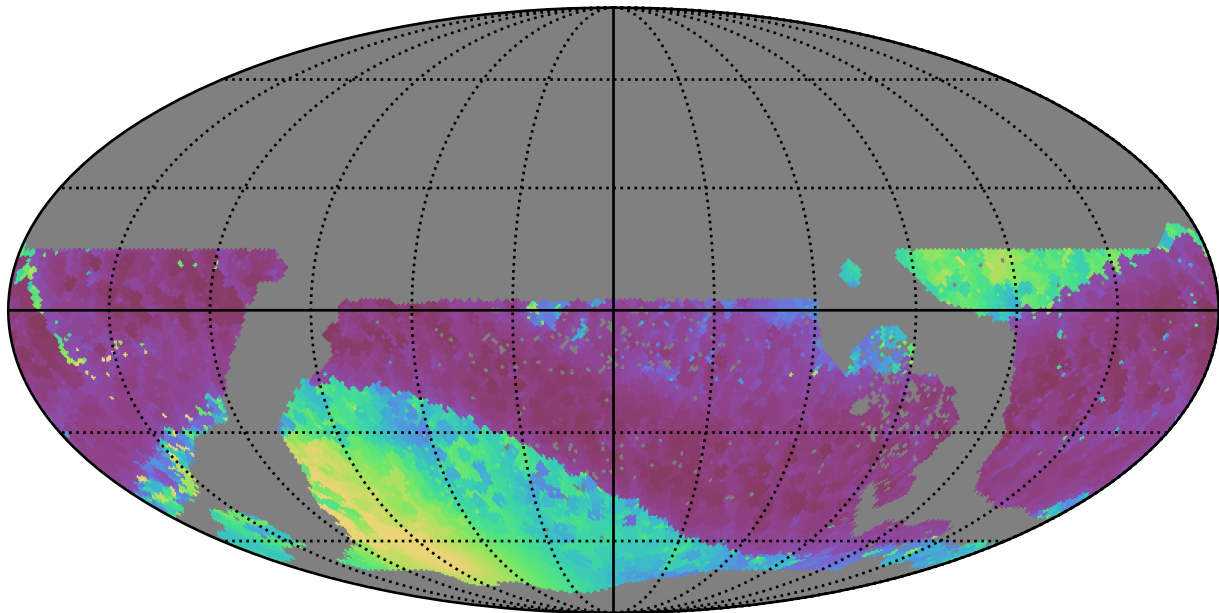
weather_cloudso0v3.4_10yrs WFD z band: Min solarElong
