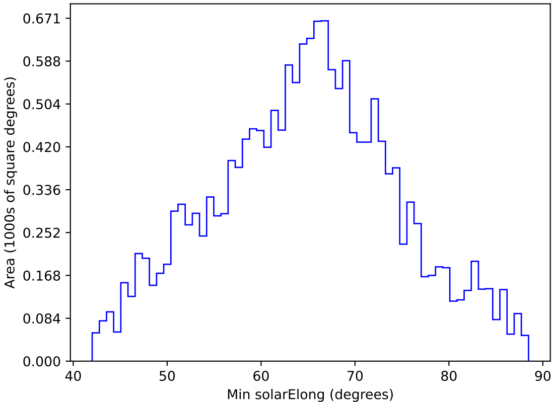
weather_cloudso0v3.4_10yrs WFD y band: Min solarElong
