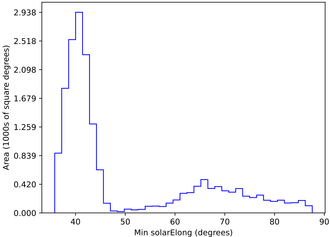
weather_cloudso0v3.4_10yrs WFD i band: Min solarElong
