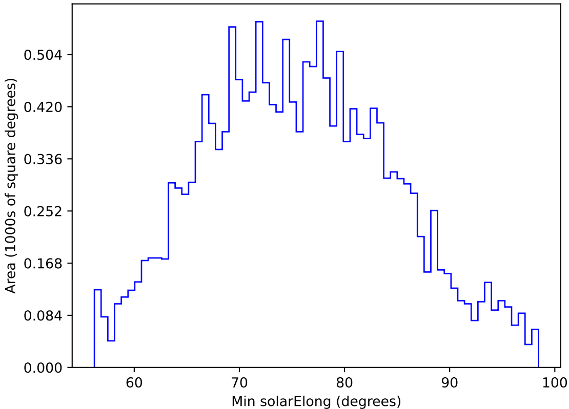
weather_cloudso0v3.4_10yrs WFD g band: Min solarElong
