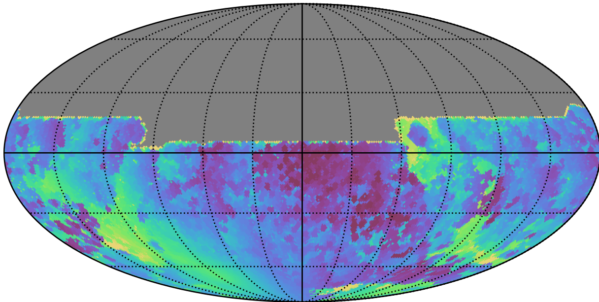
weather_cloudso0v3.4_10yrs All sky y band: Min solarElong
