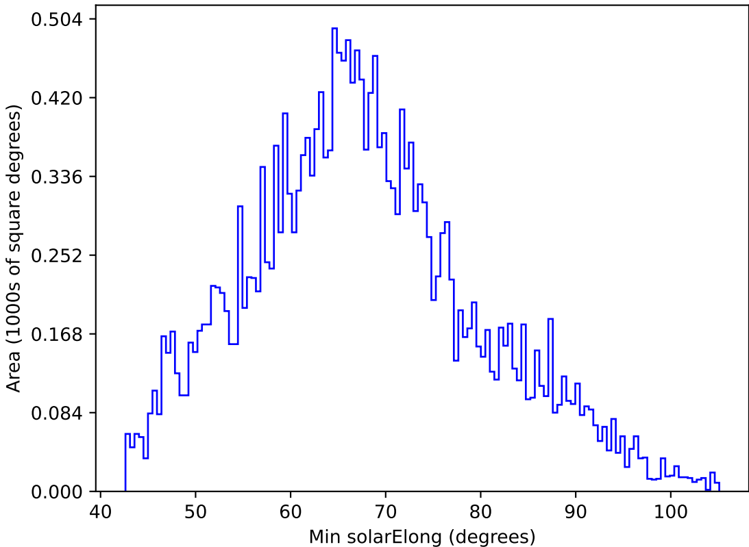
weather_cloudso0v3.4_10yrs All sky y band: Min solarElong
