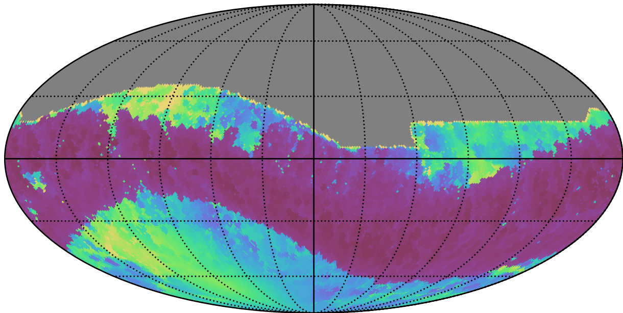
weather_cloudso0v3.4_10yrs All sky i band: Min solarElong
