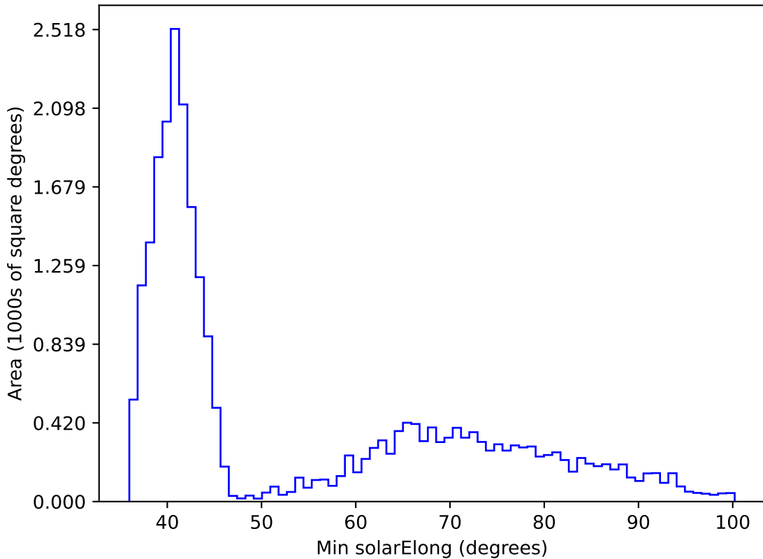
weather_cloudso0v3.4_10yrs All sky i band: Min solarElong
