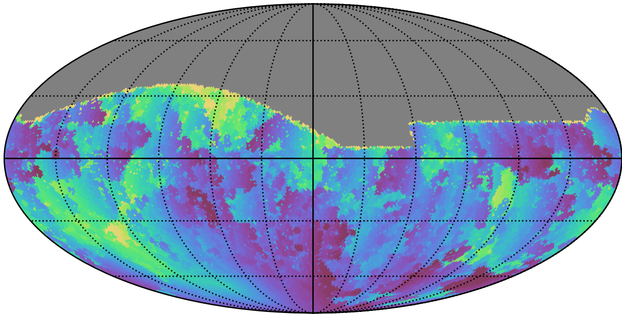
weather_cloudso0v3.4_10yrs All sky g band: Min solarElong
