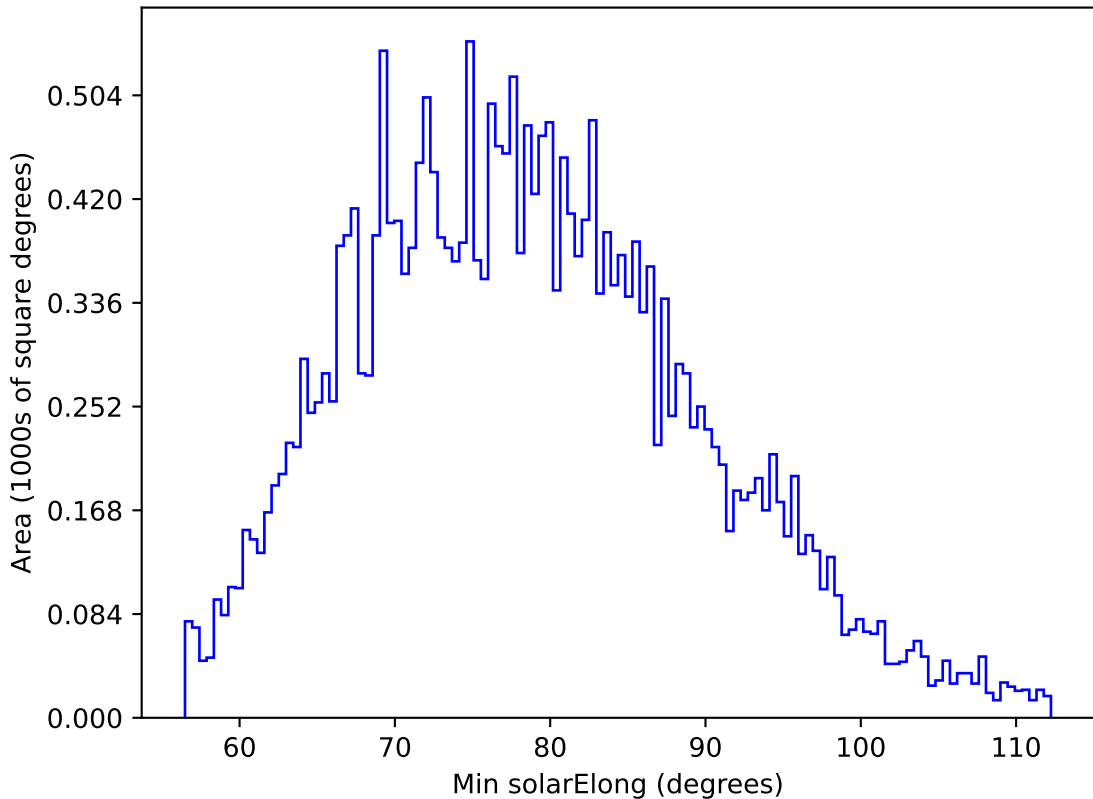
weather_cloudso0v3.4_10yrs All sky g band: Min solarElong
