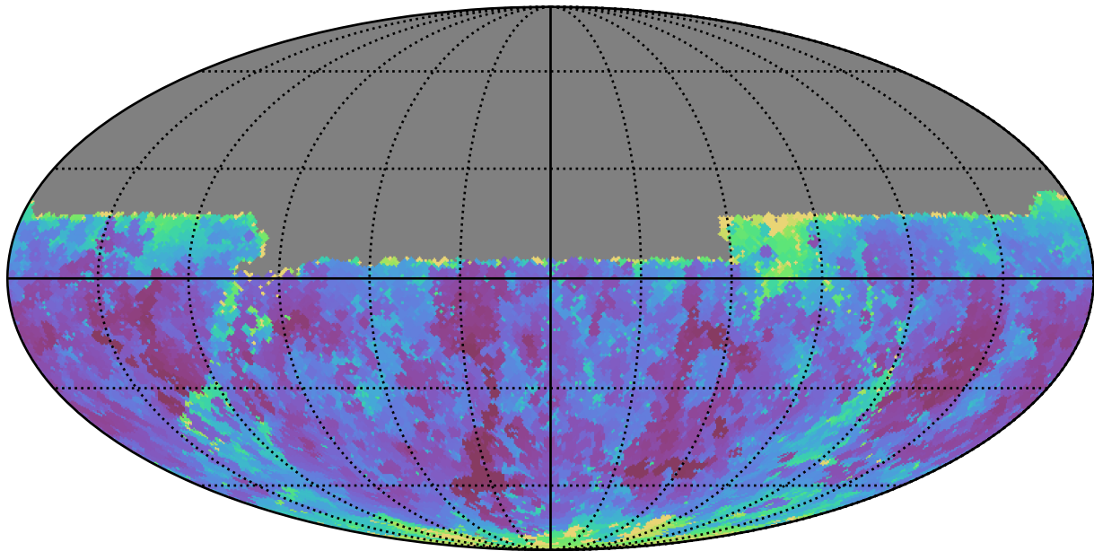
weather_cloudso0v3.4_10yrs Yr 1 y band: Min seeingGeom
