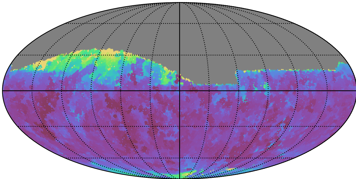
weather_cloudso0v3.4_10yrs Yr 1 i band: Min seeingGeom
