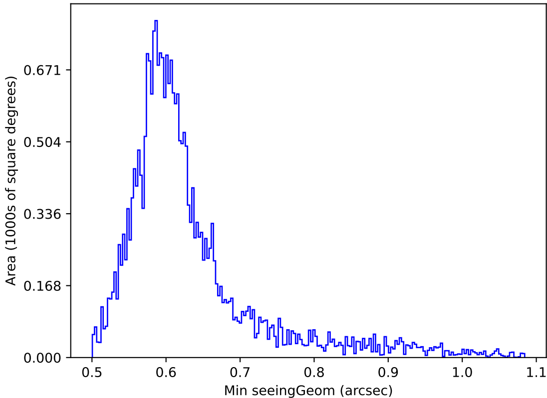
weather_cloudso0v3.4_10yrs Yr 1 i band: Min seeingGeom
