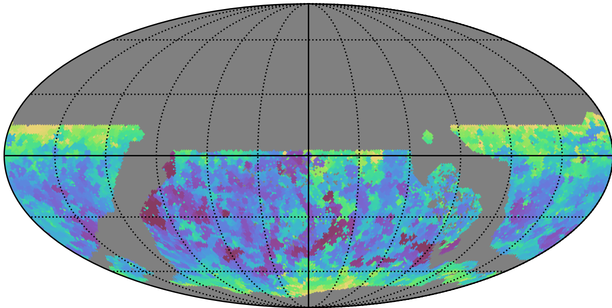
weather_cloudso0v3.4_10yrs WFD y band: Min seeingEff
