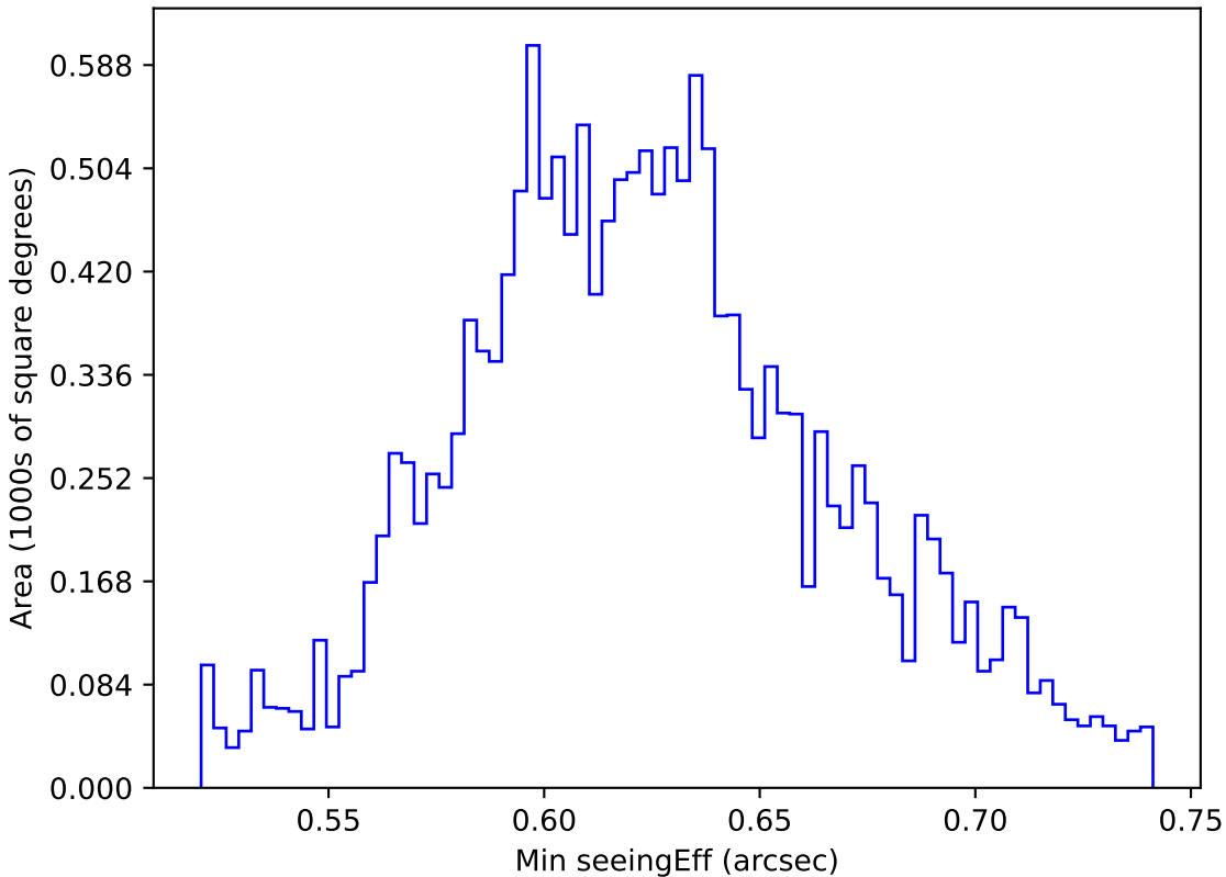
weather_cloudso0v3.4_10yrs WFD y band: Min seeingEff
