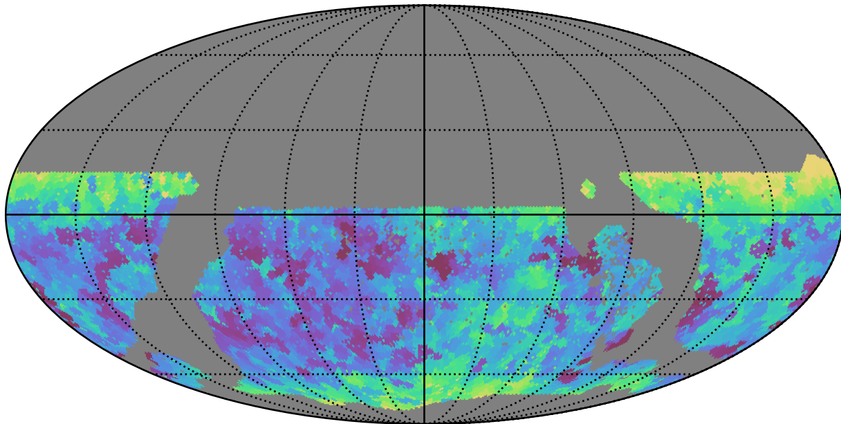
weather_cloudso0v3.4_10yrs WFD i band: Min seeingEff
