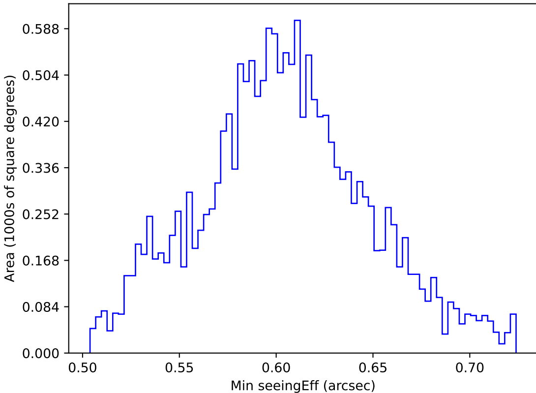
weather_cloudso0v3.4_10yrs WFD i band: Min seeingEff
