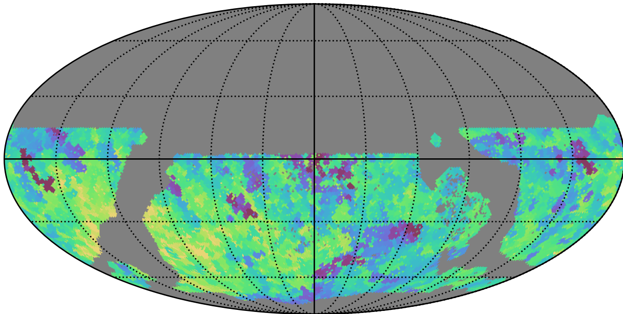
weather_cloudso0v3.4_10yrs WFD z band: Min saturation_mag
