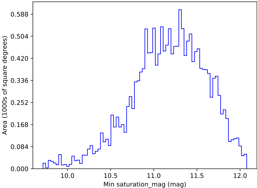
weather_cloudso0v3.4_10yrs WFD y band: Min saturation_mag
