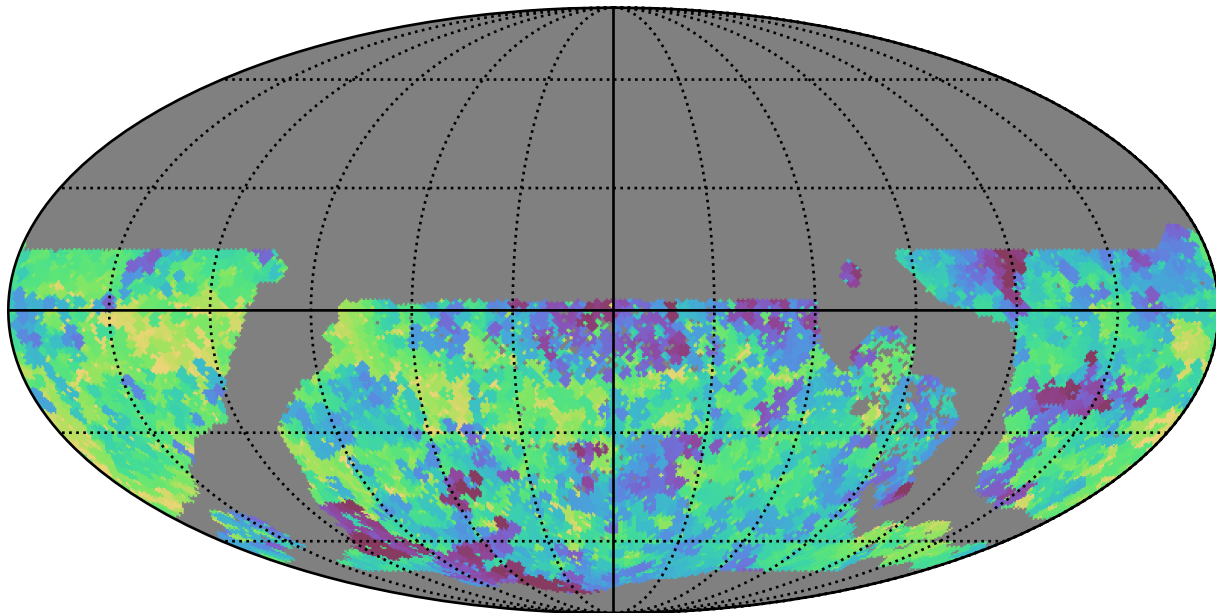
weather_cloudso0v3.4_10yrs WFD u band: Min saturation_mag
