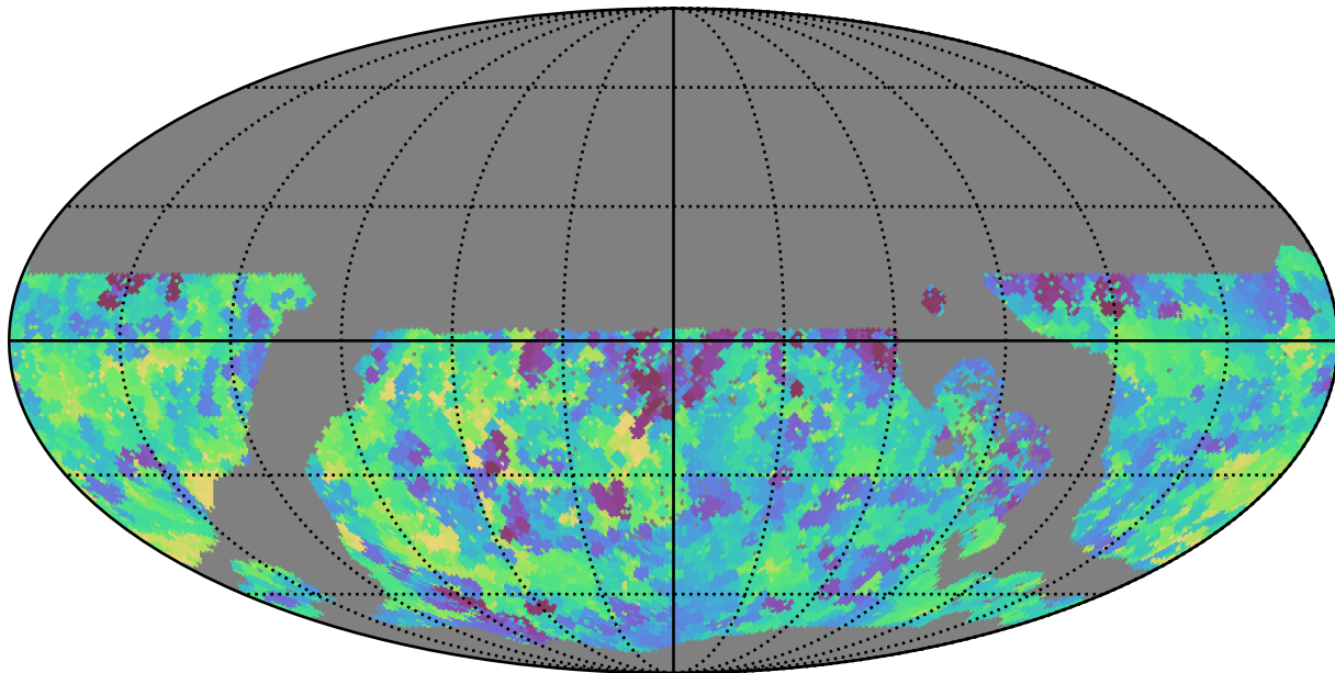
weather_cloudso0v3.4_10yrs WFD r band: Min saturation_mag
