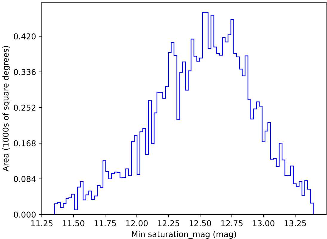
weather_cloudso0v3.4_10yrs WFD r band: Min saturation_mag
