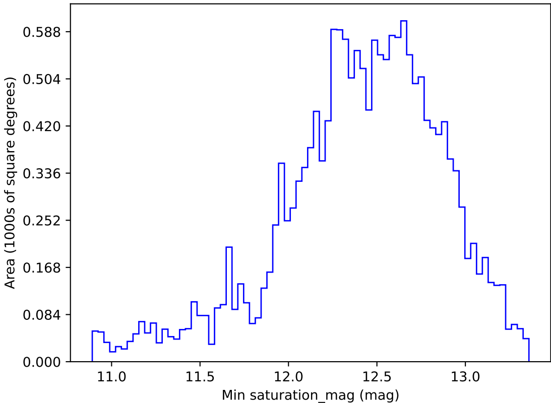
weather_cloudso0v3.4_10yrs WFD i band: Min saturation_mag
