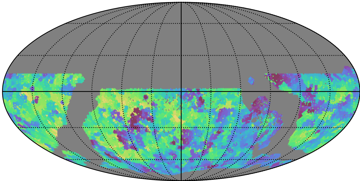
weather_cloudso0v3.4_10yrs WFD g band: Min saturation_mag
