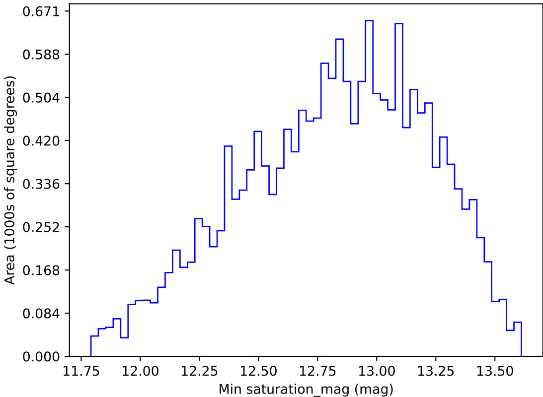
weather_cloudso0v3.4_10yrs WFD g band: Min saturation_mag
