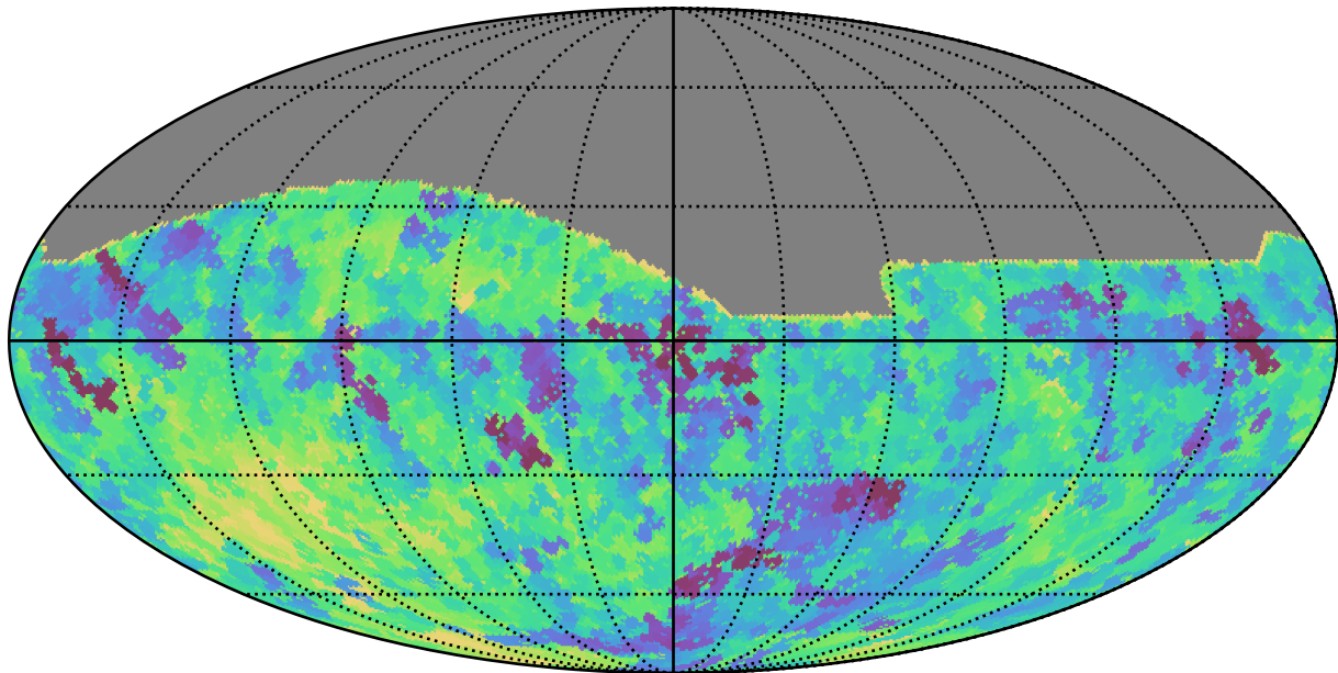
weather_cloudso0v3.4_10yrs All sky z band: Min saturation_mag
