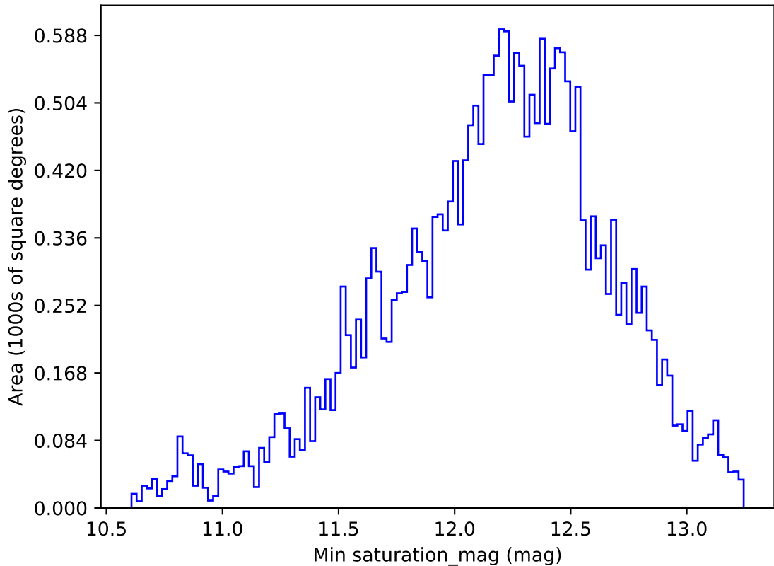
weather_cloudso0v3.4_10yrs All sky z band: Min saturation_mag
