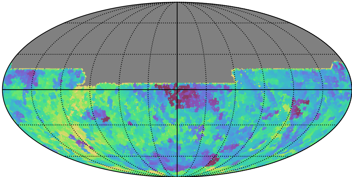
weather_cloudso0v3.4_10yrs All sky y band: Min saturation_mag
